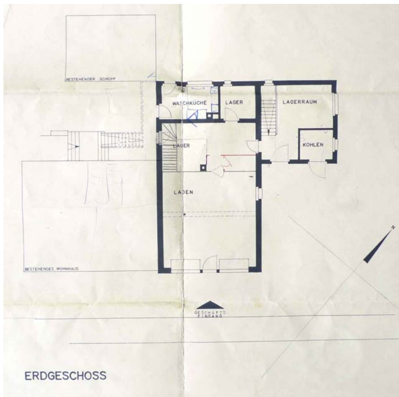
Grundriss Erdgeschoss (2012, im Besitz der Eigentümer)
