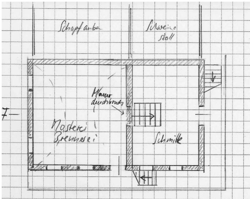
Grundrisskizze Erdgeschoss (1992)
