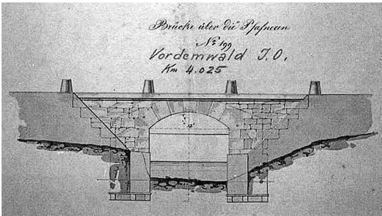
Projekt Gatschet, Ansicht und Schnitt (aus: IVS AG 359.2.1)
